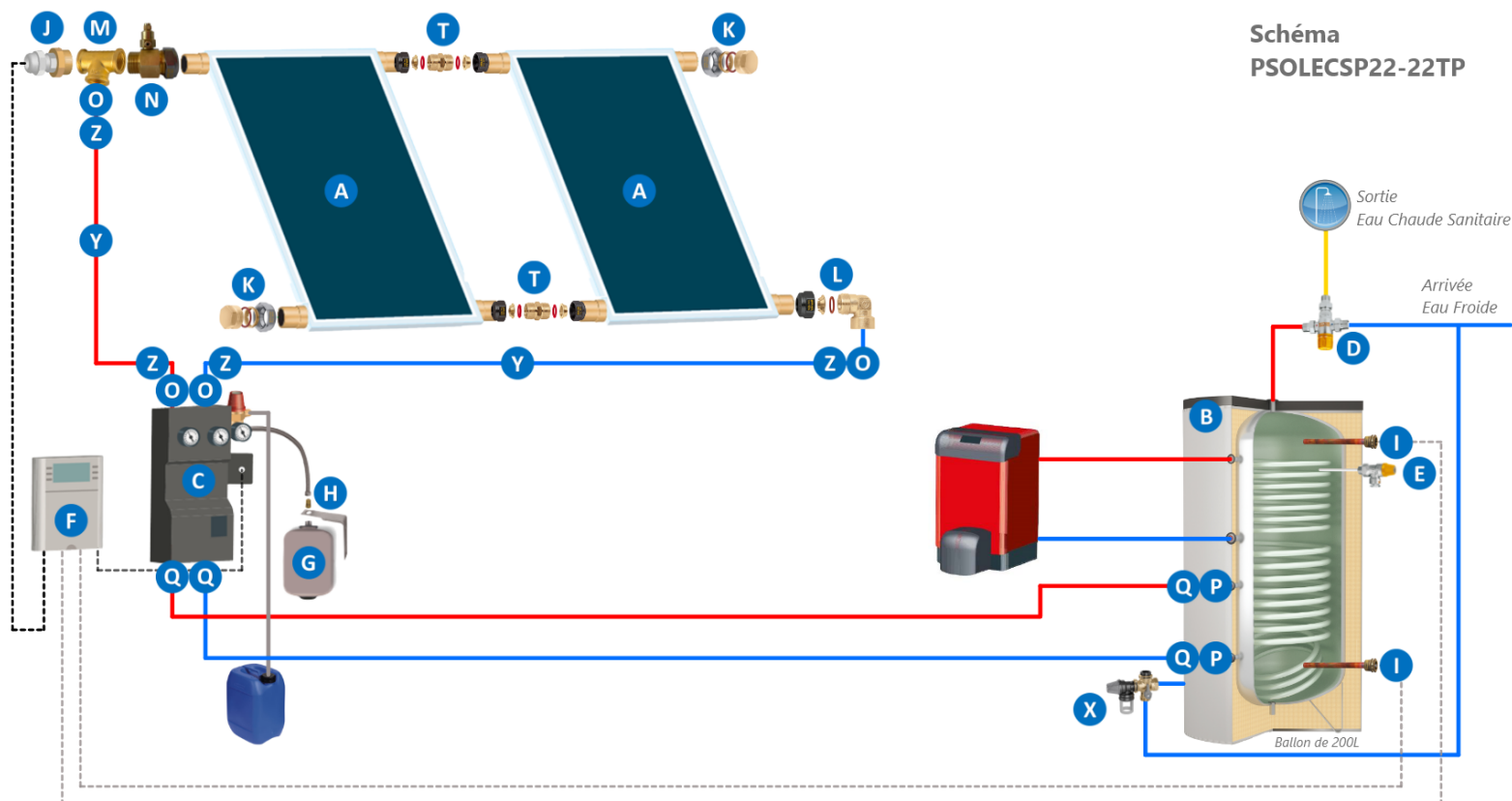
Nomenclature PSOLECSP22-22TP
