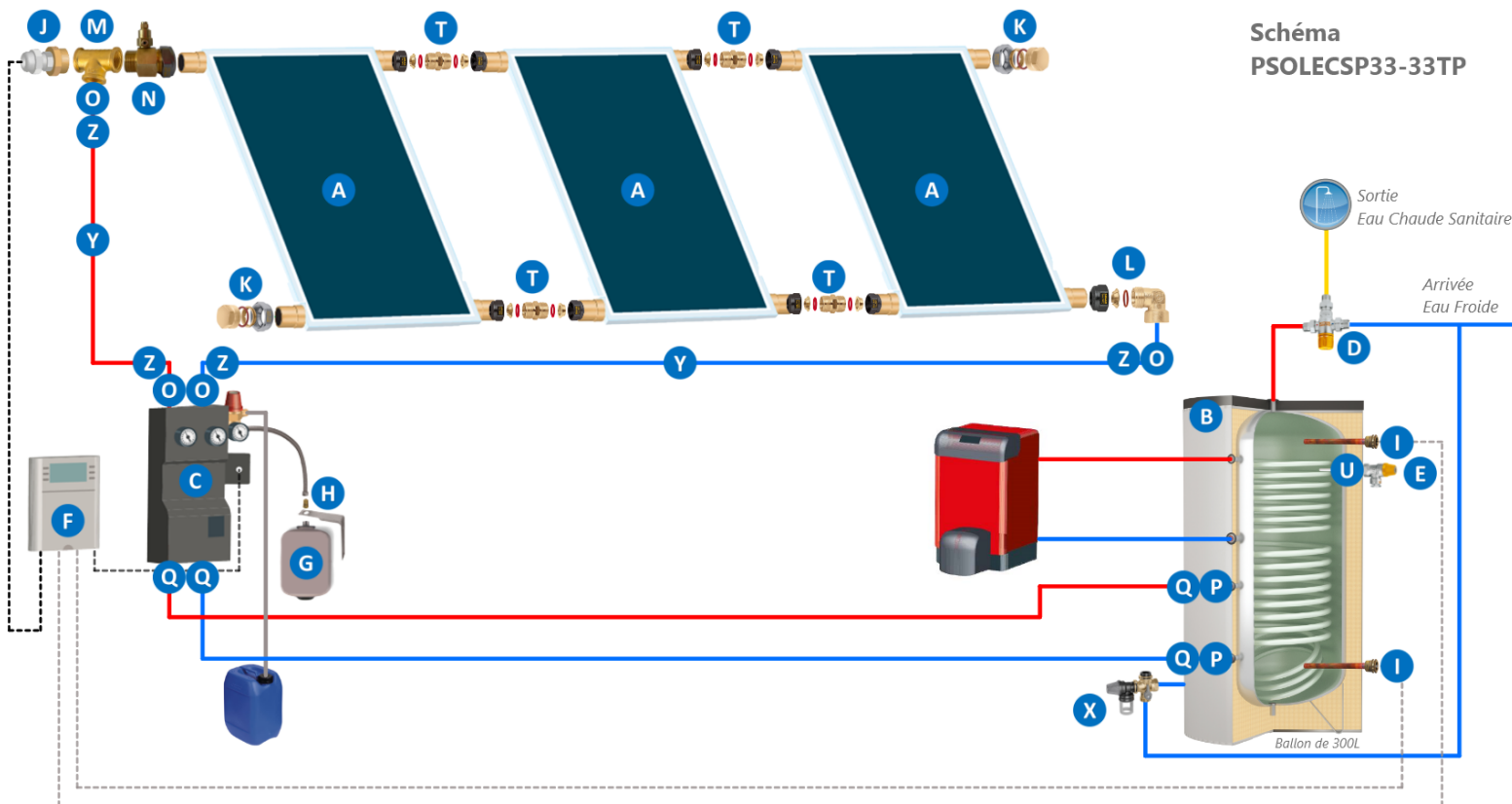
Nomenclature PSOLECSP33-33TP
